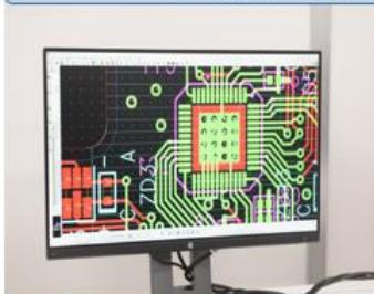
基板設計
