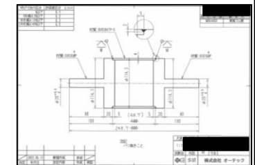
[自社設計図]
