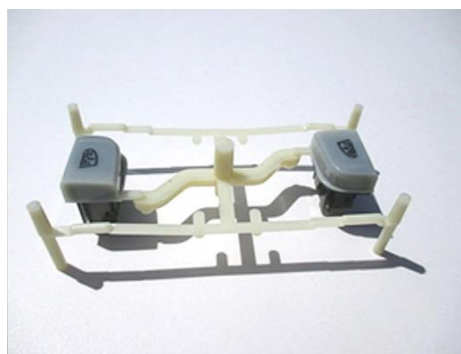
2色成形用金型
